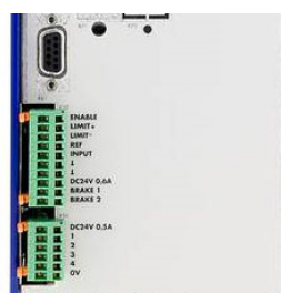
JetMove JM-215
